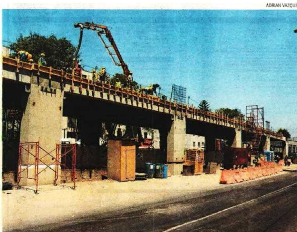
Avance de la Calzada Elevada sobre Tlalpan obra que construye el Gobierno de la CDMX por la Copa Mundial
